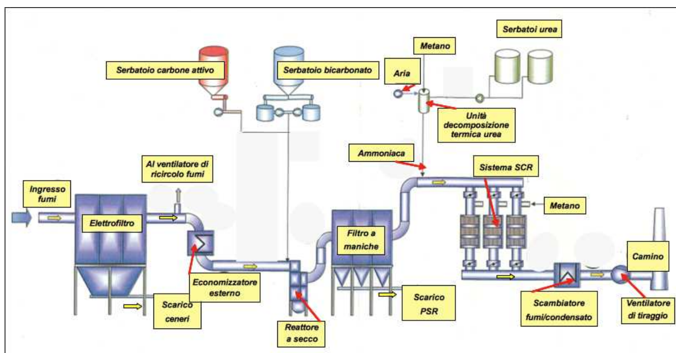
Fig. 6 Schema dell'impianto di trattamento fumi (tratto dal sito www.trm.it )
