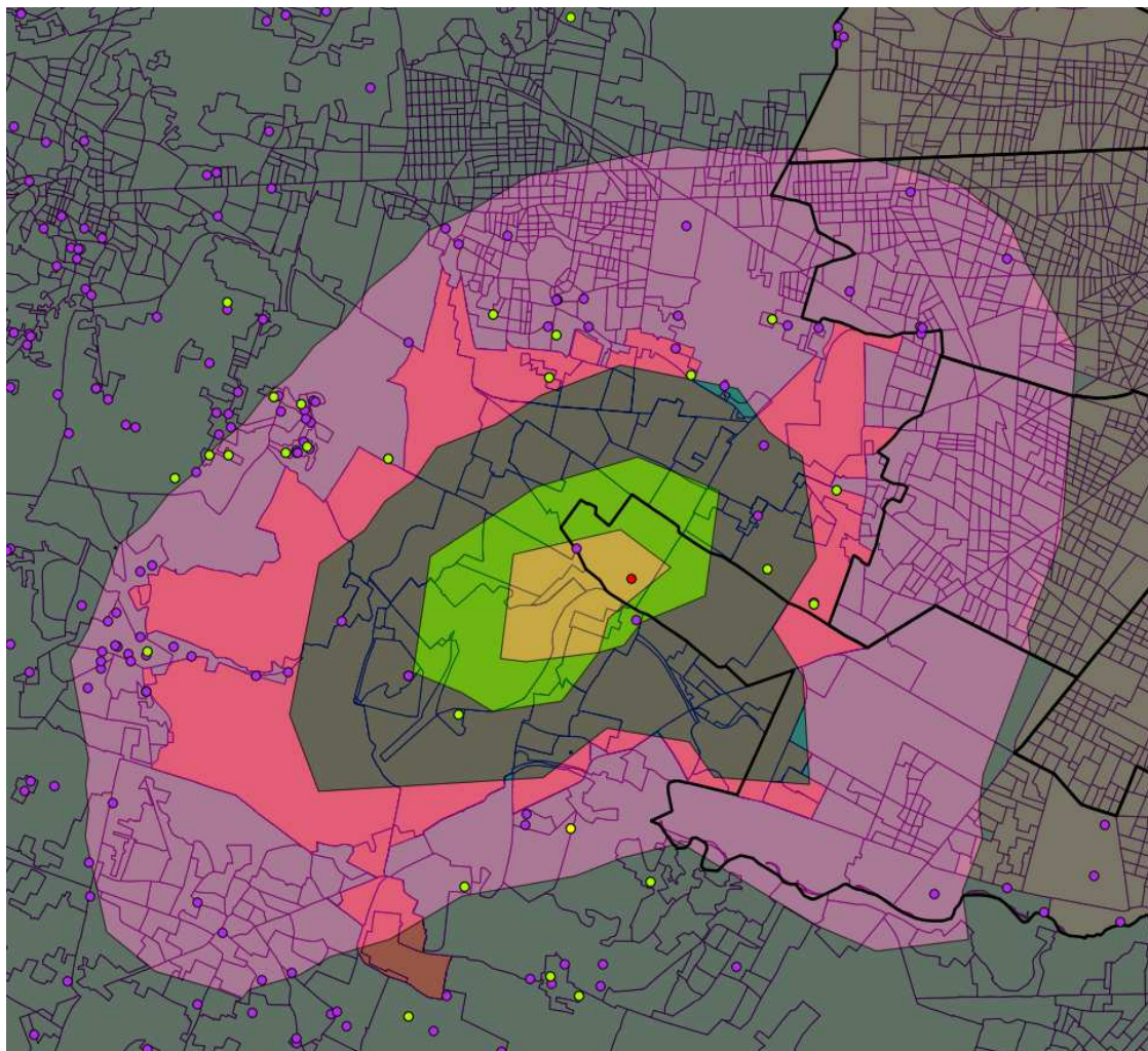
Fig. 6 Aree di ricaduta nelle zone circostanti l'inceneritore (rappresentato con un cerchio rosso). In viola sono rappresentati gli allevamenti presenti in ARVET e in verde gli allevamenti selezionati per il monitoraggio biologico.
